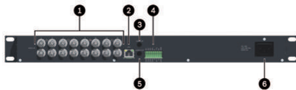
Fig. 3: VIDEOJET multi 4000 rear
